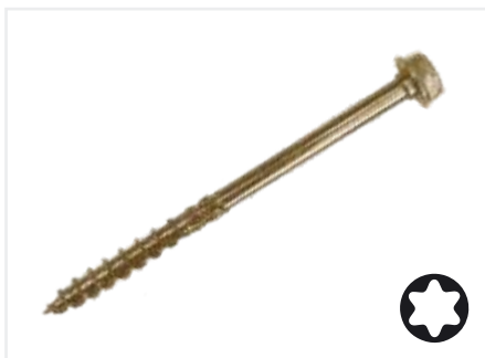
Șurub de construcții cu cap hexagonal și guler amprentă torx, cu freză la mijloc și amprentă tip 17
