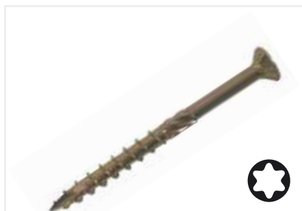
Șurub de construcții cu cap înecat, amprentă torx, cu freză la mijloc și vârf tip 17
