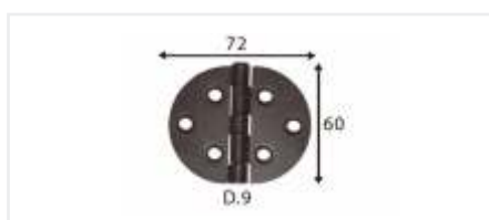
Balama pafta cu aripi rotunjite, tip 1 brunată (mm)
