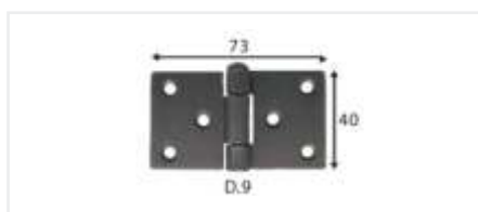
Balama dreptunghiulară, tip 1 brunată (mm)
